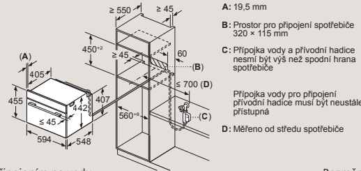
CS9... s připojením na vodu
